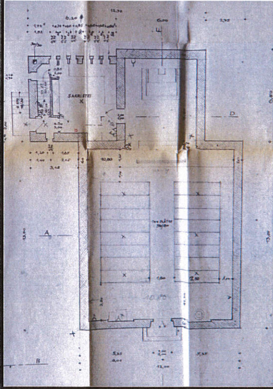
Ursprünglicher Grundriss der Kapelle aus den Bauantragsunterlagen mit Darstellung der Ausstattungsdisposition. (LWL-DLBW)
